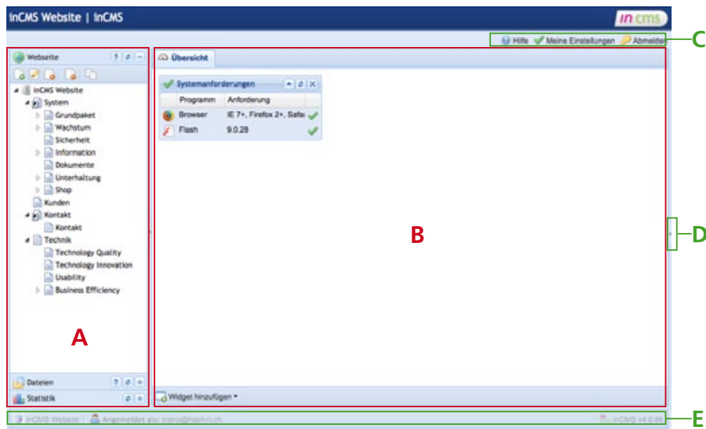
Abb. 1: Die inCMS-Benutzeroberfläche
